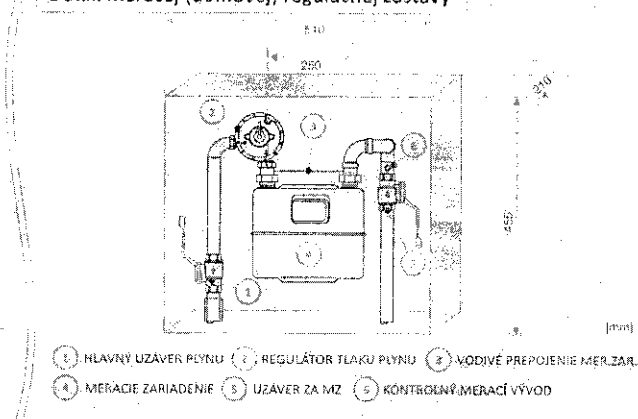
Detail meracej (domovej) regulačnej zostavy
